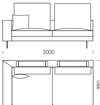
Siedzisko 3
