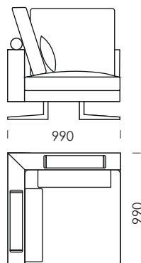
Element narożny
