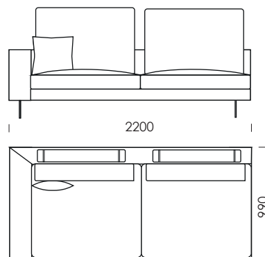
Siedzisko 4
