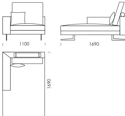
Szezlong 2
